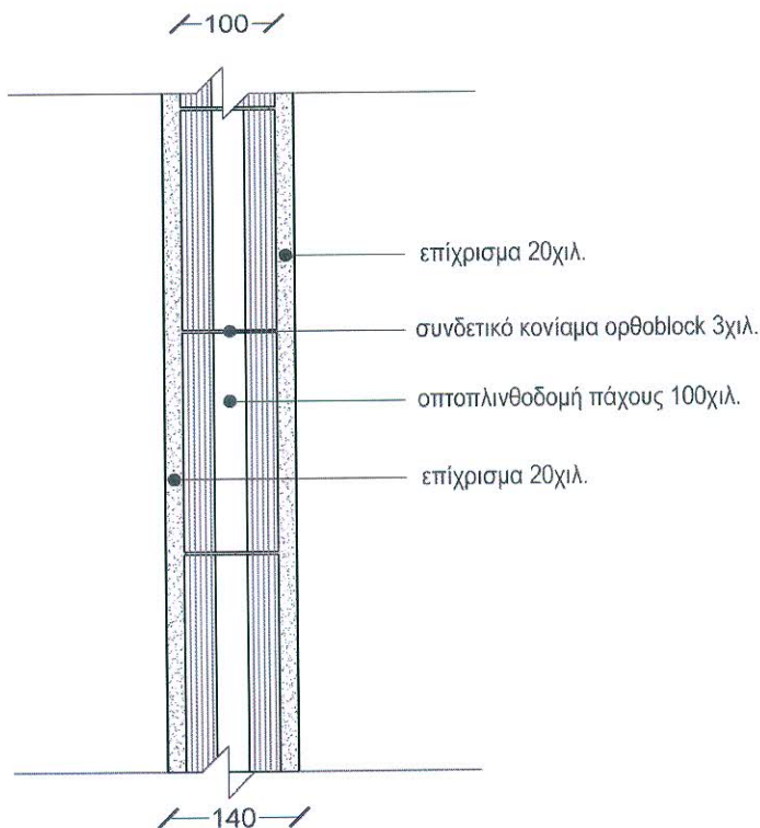
Κατακόρυφη τομή / Vertical section
