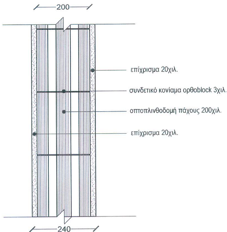
Κατακόρυφη τομή / Vertical section
