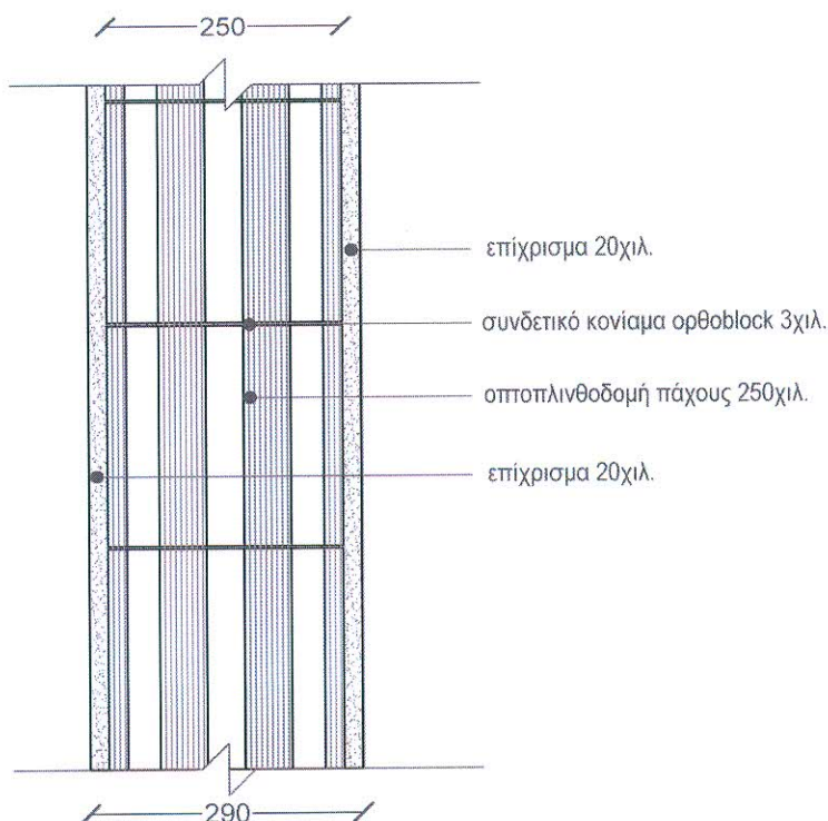
Κατακόρυφη τομή / Vertical section
